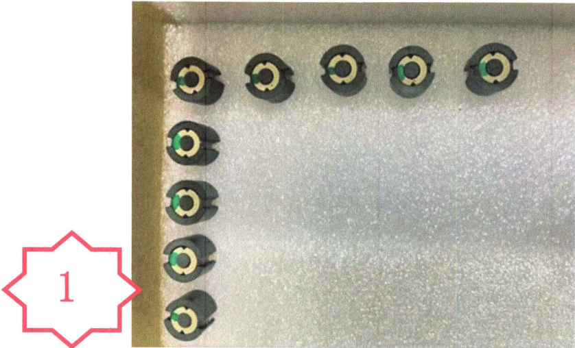
图一，将 PA05475 组件如图装入珍珠棉，一格 5 个
